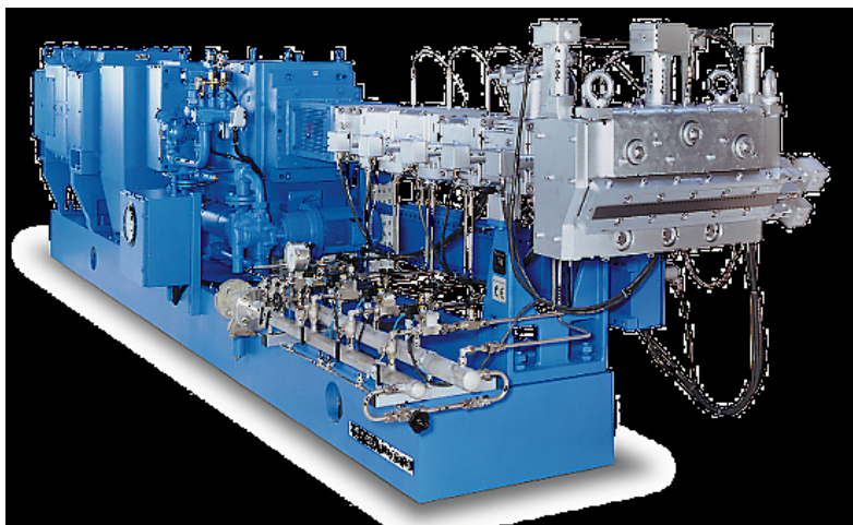
Moderner Compoundierextruder (Bild: Coperion)
